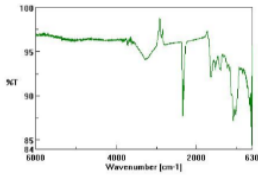
Fig.1 Cladophora Spectre IR
